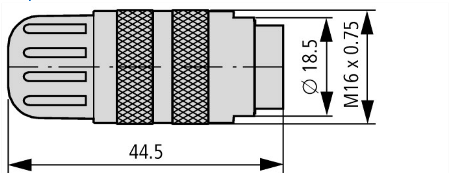
Штекерные разъемы для проводов круглого сечения SmartWire-DT, прямые
