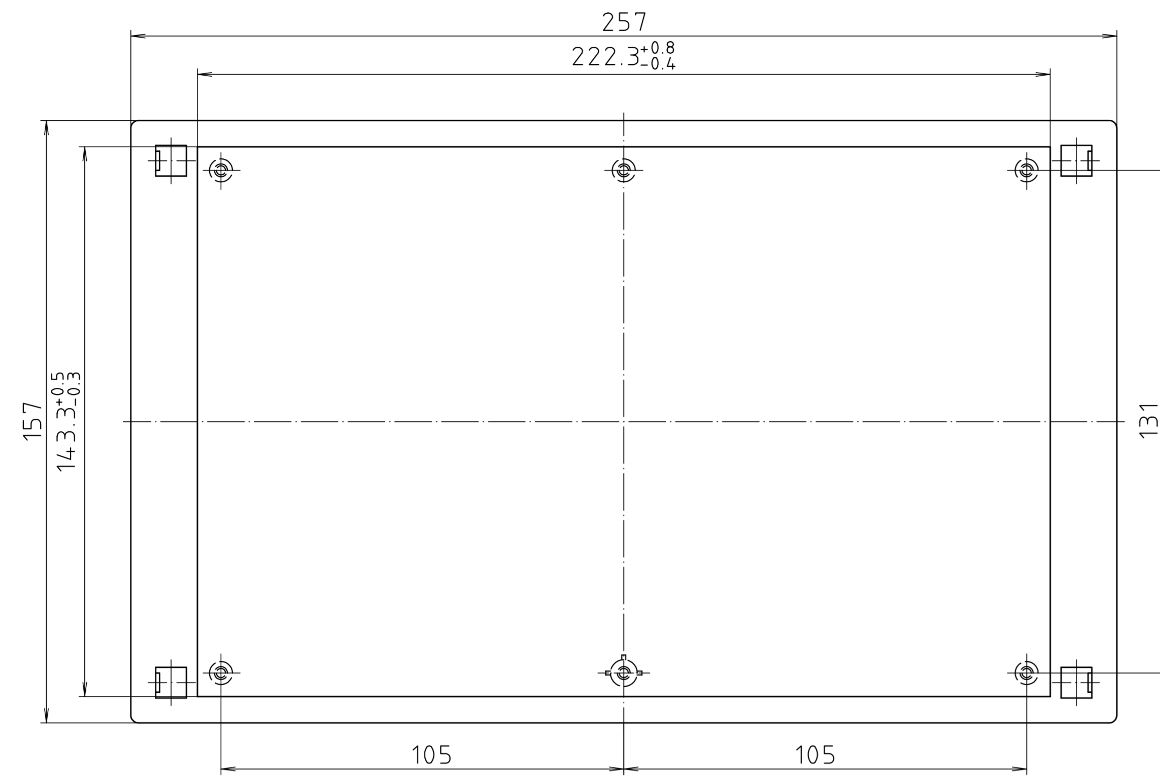
Schalttafel-ausschnitt/ panel cut-out
