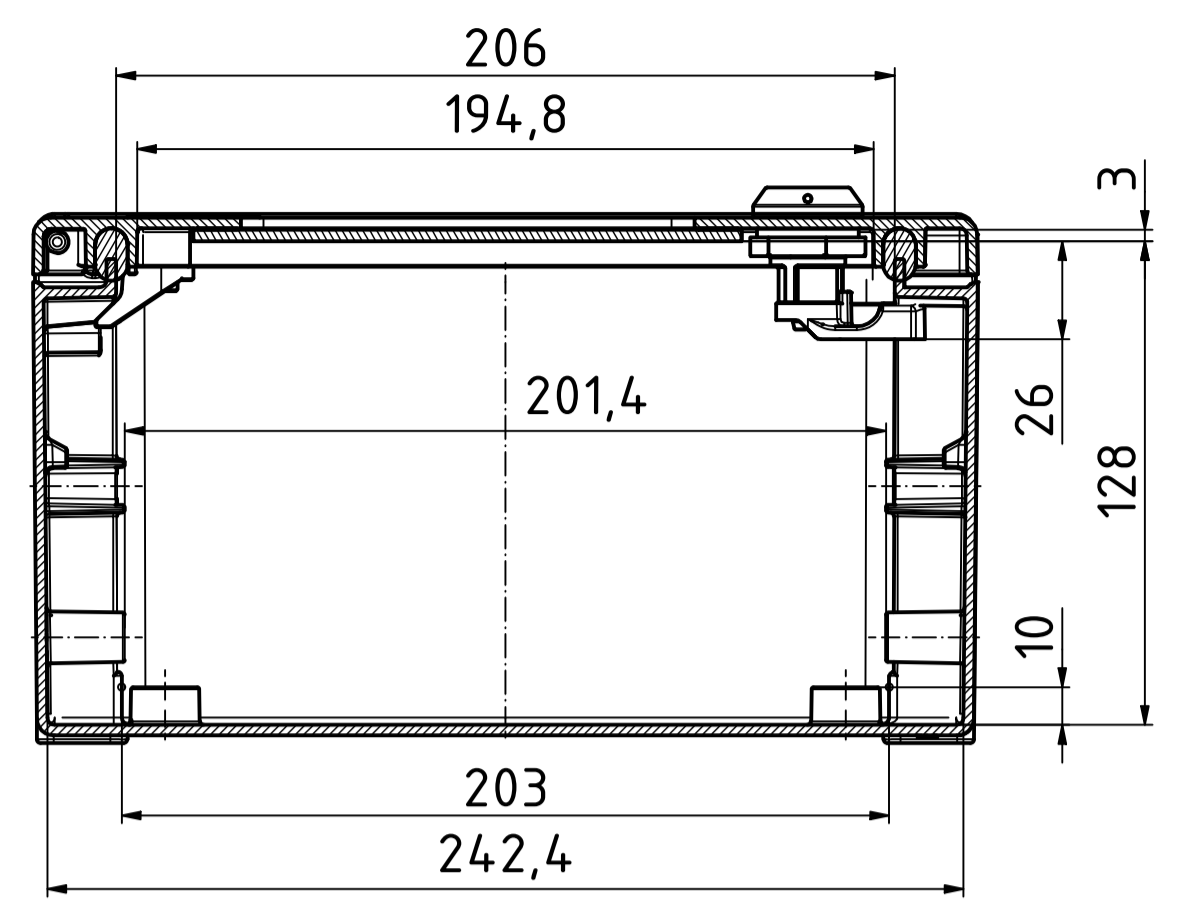
A-A ( 1 : 2 )
