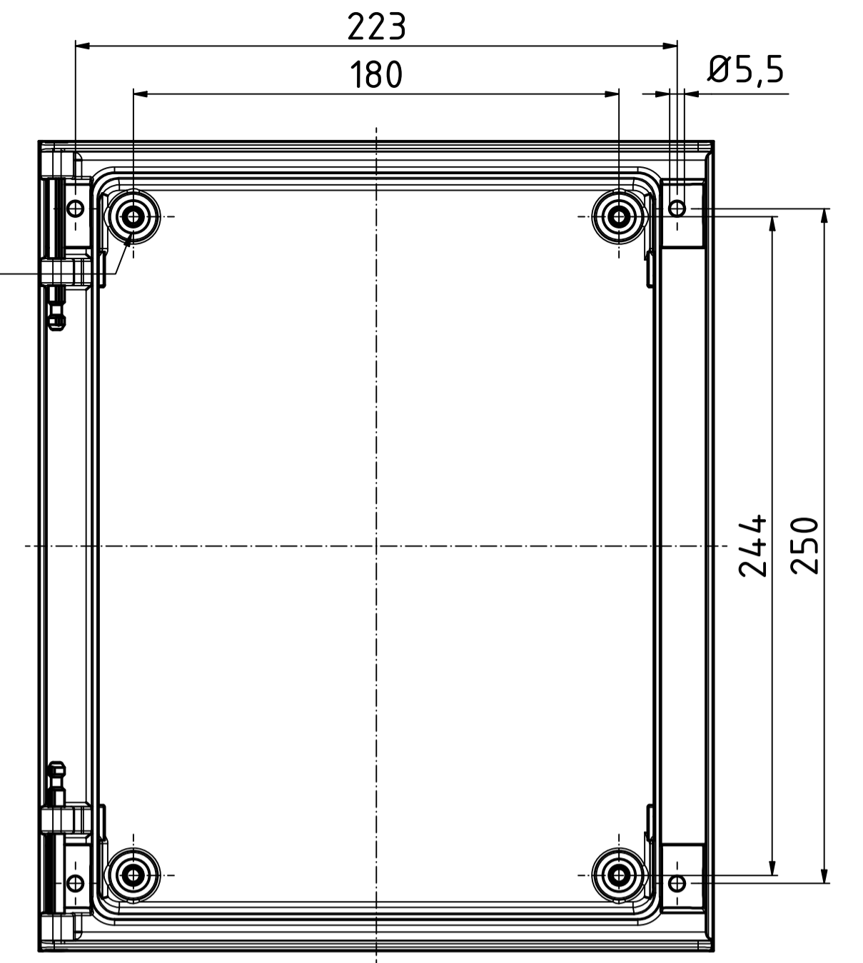
Unterteil/base ( 1 : 2 )
