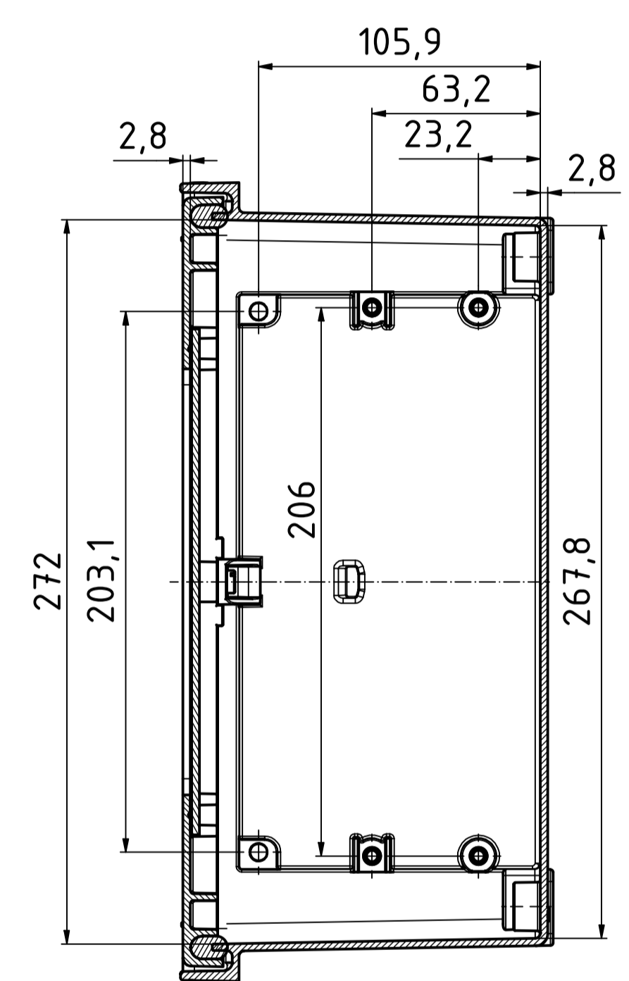
B-B ( 1 : 2 )
