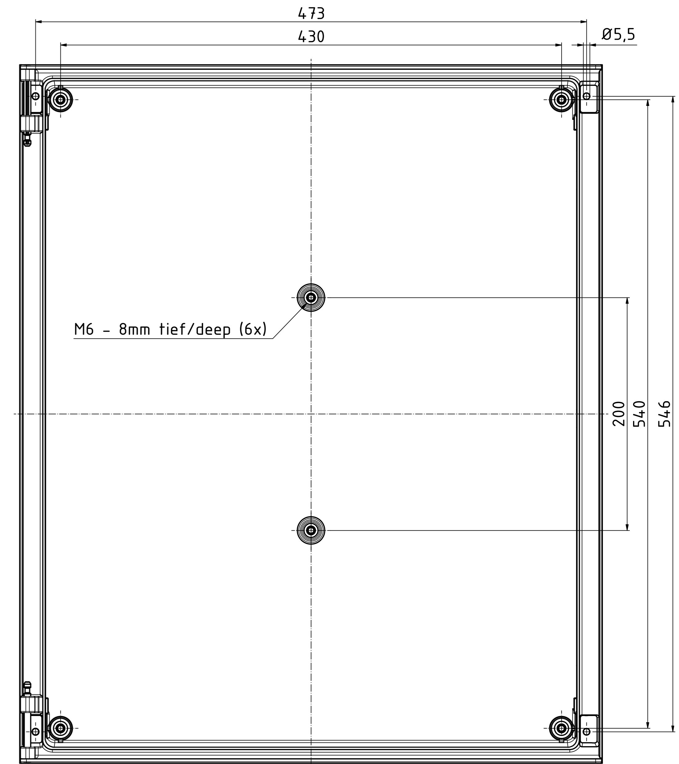
Unterteil/base ( 1 : 2 )
