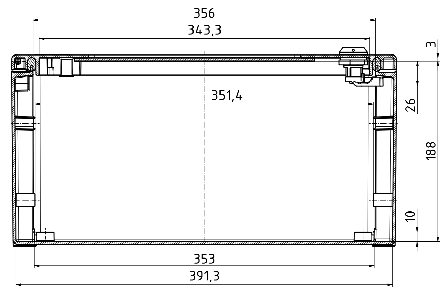
A-A ( 1 : 2 )
