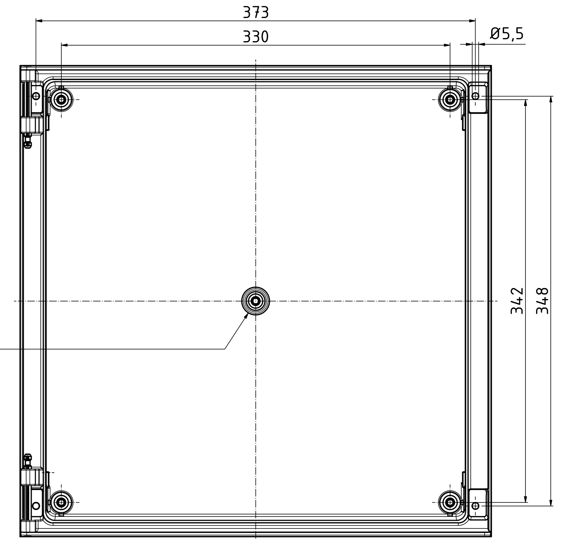
Unterteil/base ( 1 : 2 )
