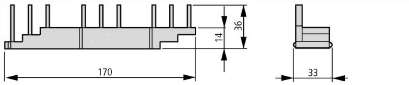
Шинный соединитель трехфазного тока
