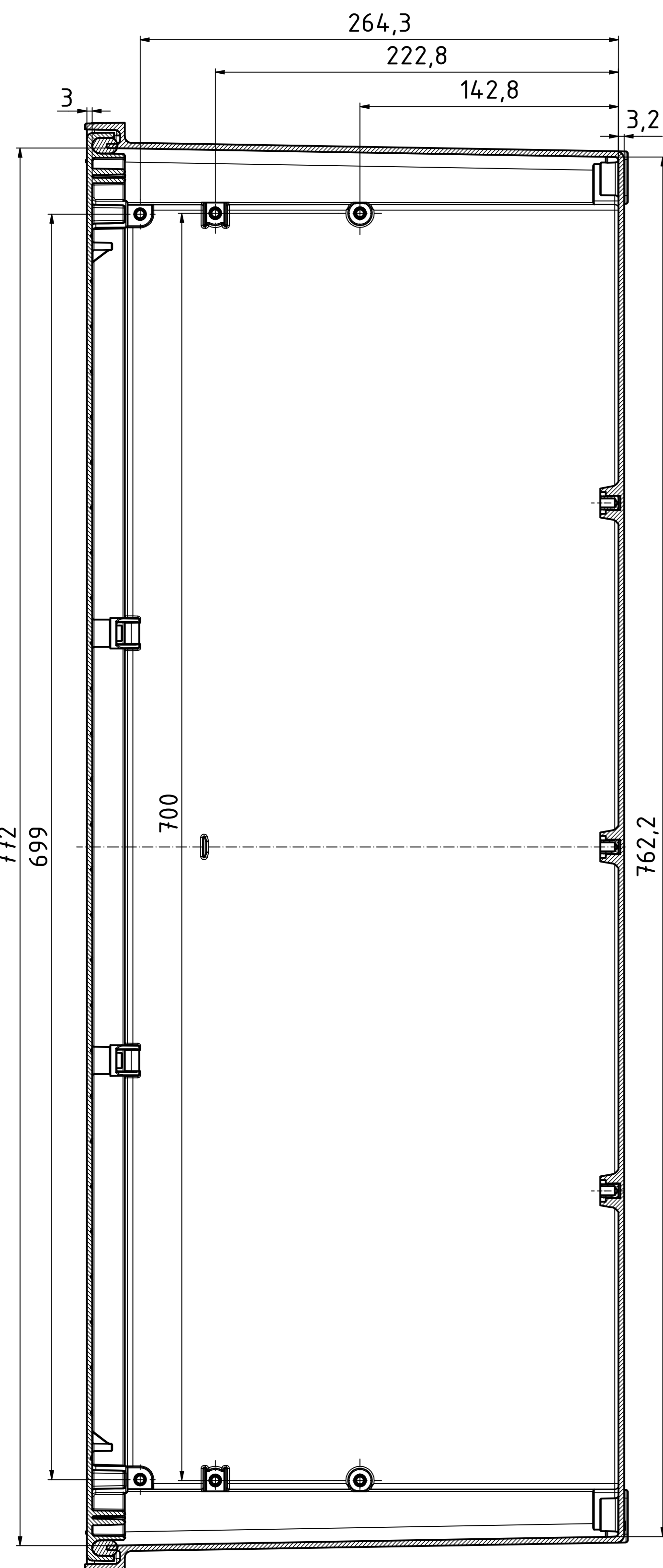
B-B ( 1 : 2 )
