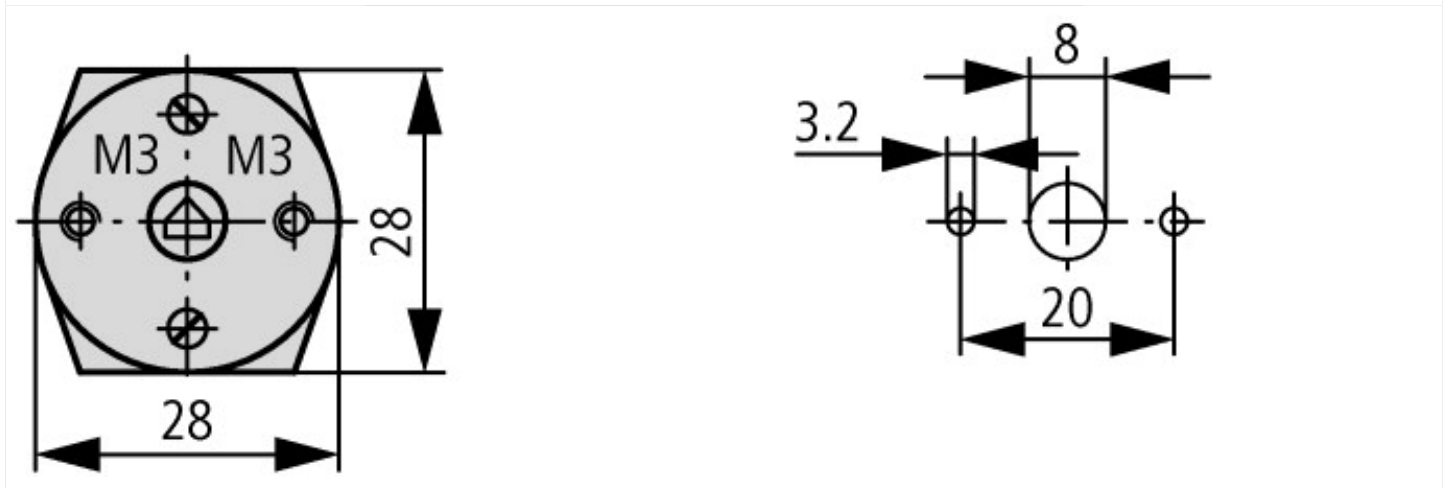
Шаблоны сверления для двери
