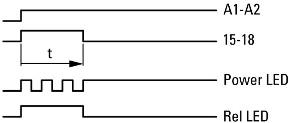
42 мигание, с началом импульса
