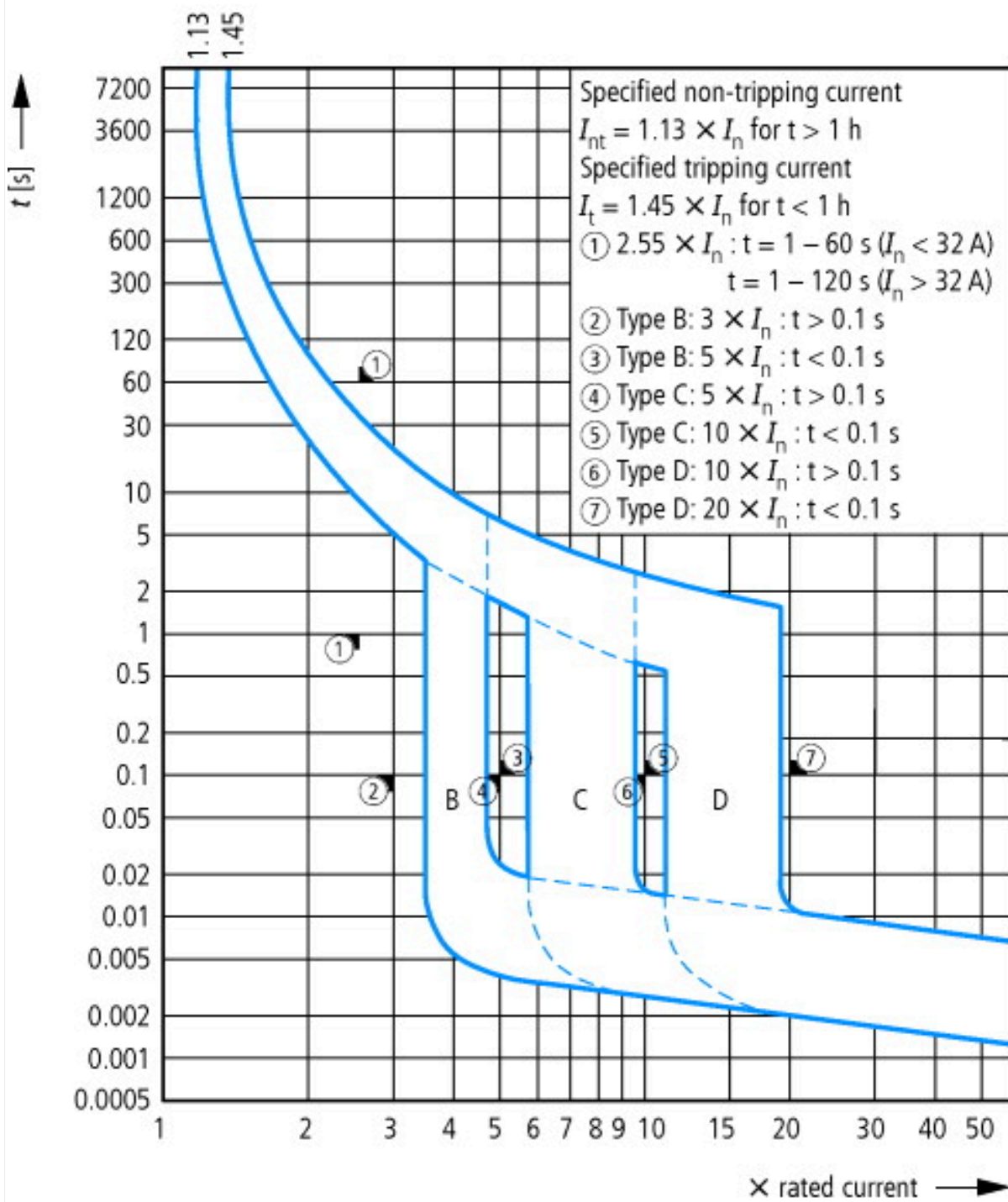
Характеристика срабатывания при 30 °C: Замыкающий контакт согласно IEC/EN 60947
