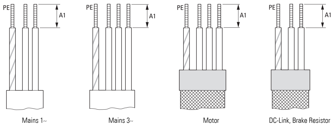
Abbildung 43: Abisolierlängen im Leistungsteil
