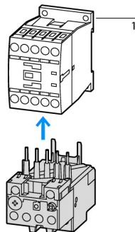
1 Силовые контакторы
