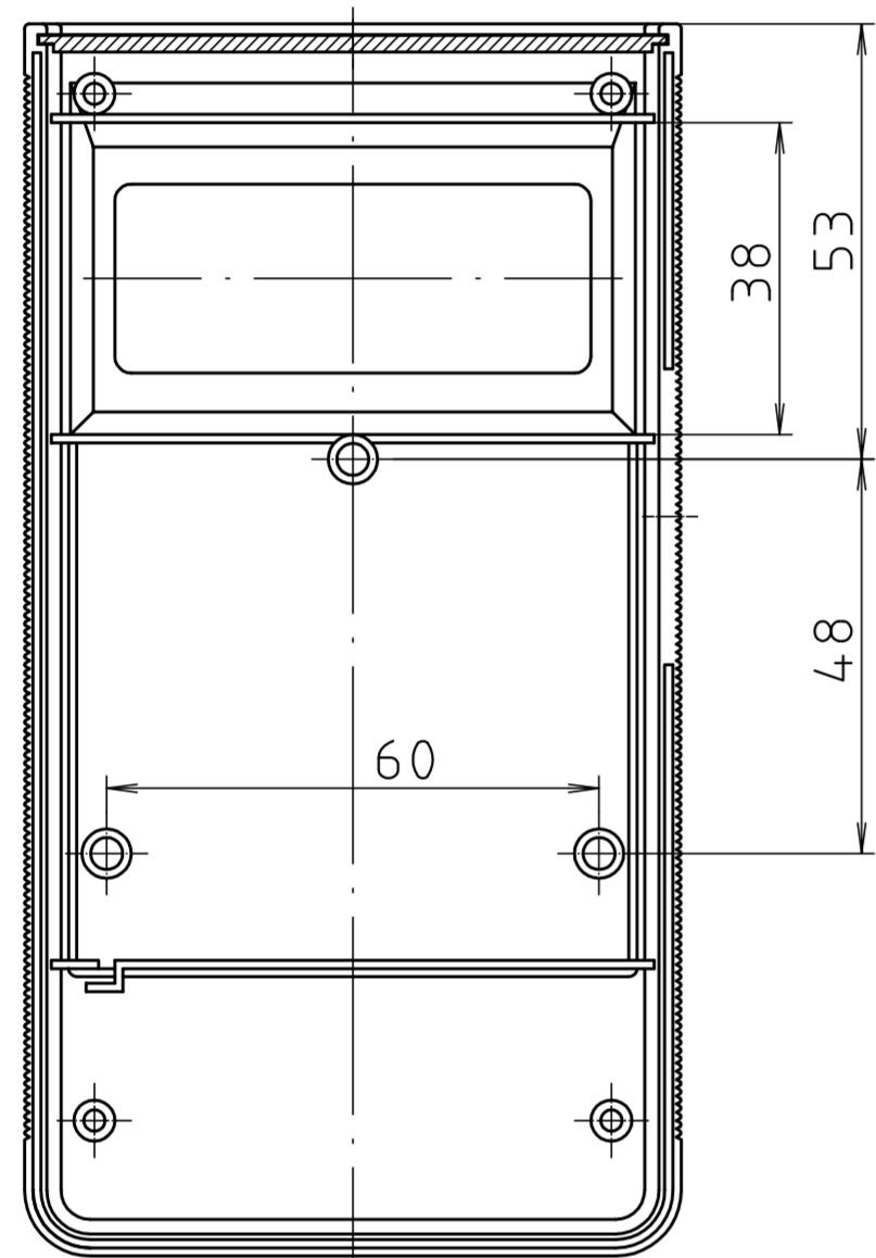
Oberteil von Innen/ Lid inside
