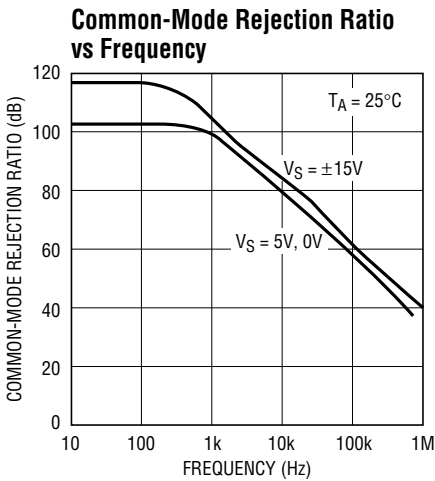
LT1413 • TA15
