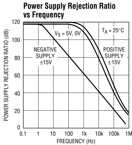
LT1413 • TA16
