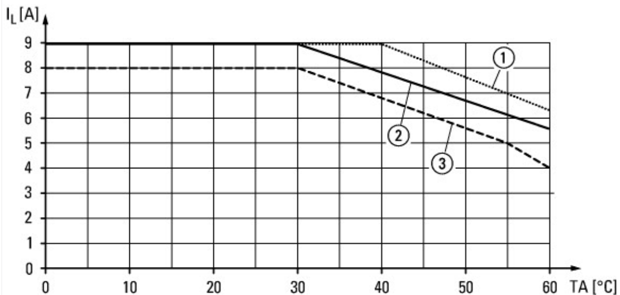
Характеристика расщепления КЛАСС 10A настроенный ток двигателя > 4 А
